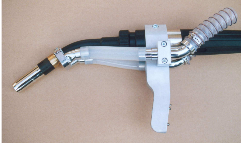
Brenner ausgerüstet mit ROPAS-Absaugdüse Typ KOMPAKT (sehr guter Erfassungsgrad)
